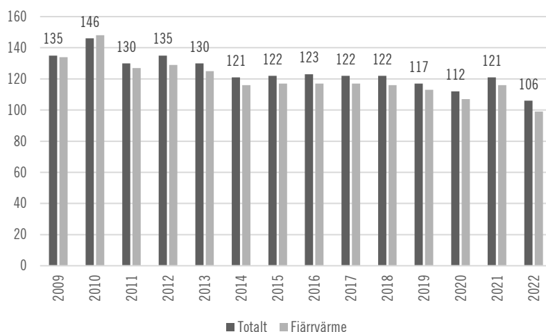
Figur 6.38 Energianvändning fördelat på uppvärmningssätt 2009–2022
