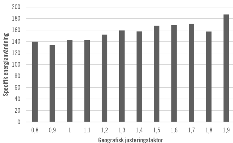
Figur 6.40 Genomsnittlig specifik energianvändning sorterat efter geografisk justering
